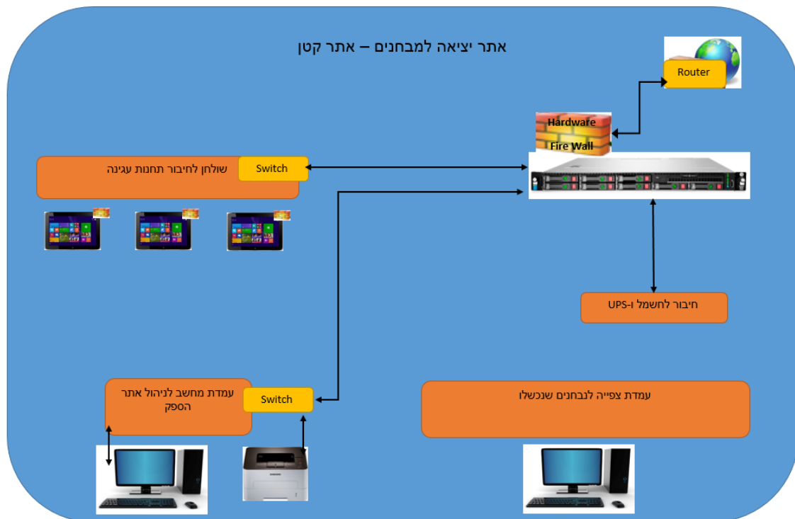
5.1.3. אתר בינוני, להלן המחשה לשרטוט סכמתי של האתר :
