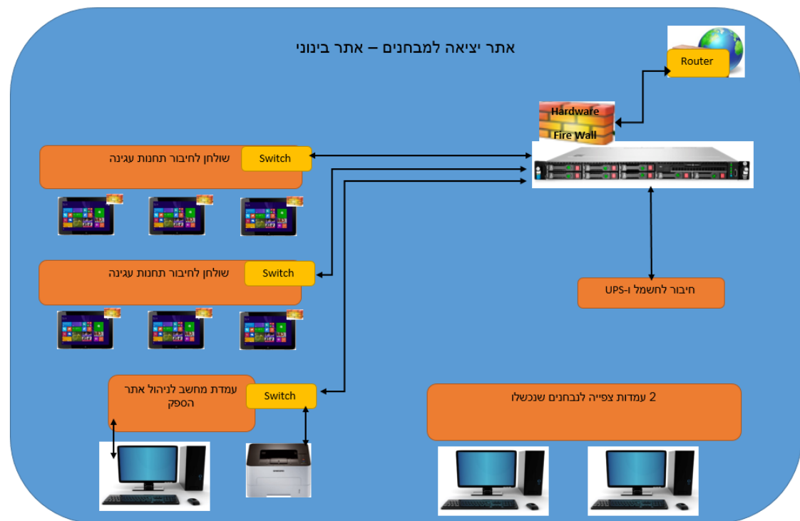
5.1.4. אתר גדול (ירושלים בלבד), להלן המחשה לשרטוט סכמתי של האתר :
